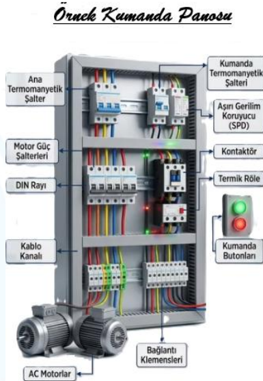
Örnek Kumanda Panosu
