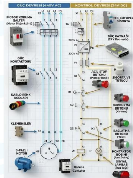
Örnek Güç ve Kontrol Devre Şeması
