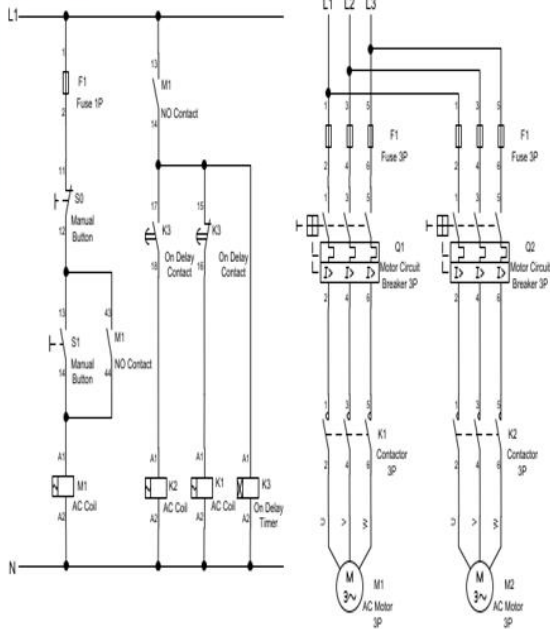
Örnek Kumanda Şeması
